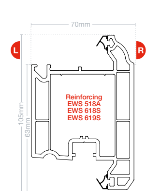
Reinforcing EWS 518A EWS 618S EWS 619S Door sash T EWS 7719
