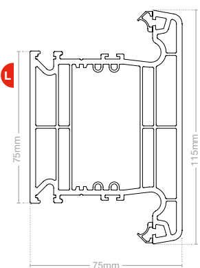
Door mid rail LSF 1009
